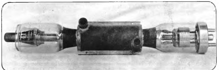
Watergekoelde Western Electric Zendlamp, vermogen 10 K.W.
